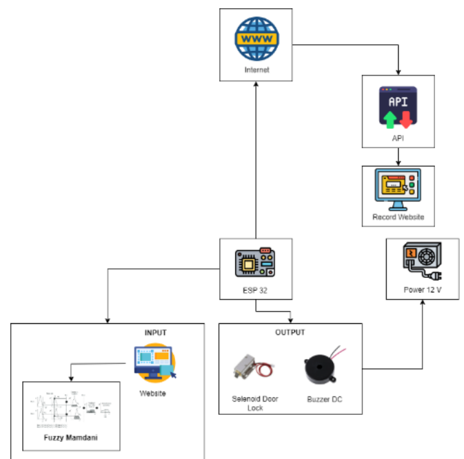
Gambar 1 Desain Sistem
